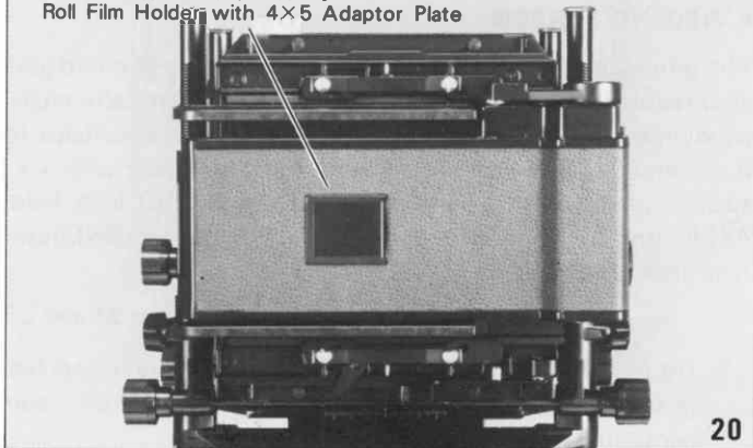
45フレーム付ロールフィルムホルダー Roll Film Holder with 4×5 Adaptor Plate
